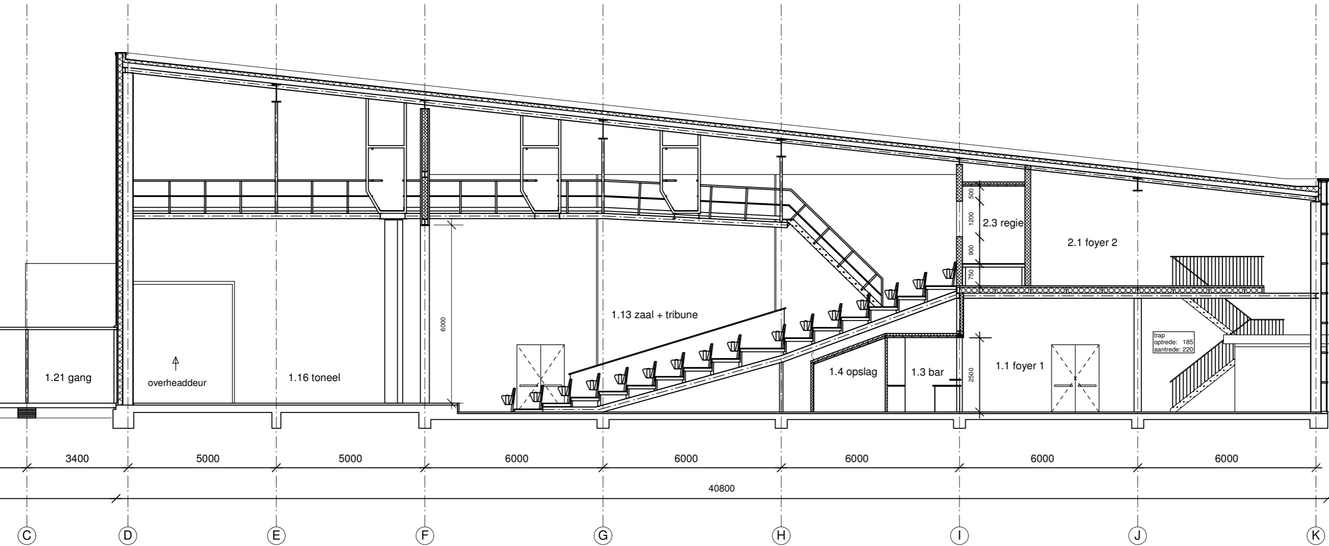
- DOORSNEDE AA' -
